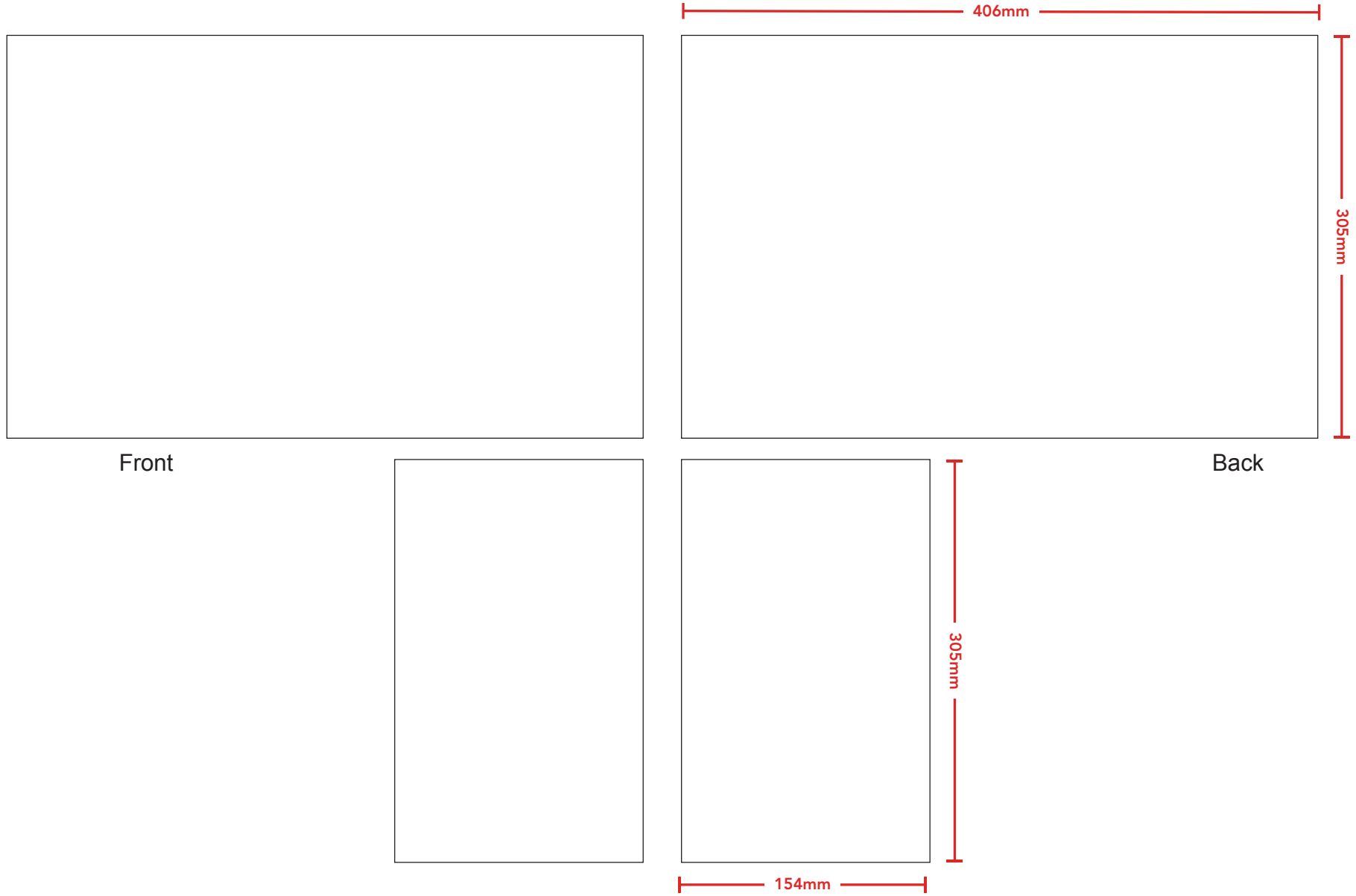
Left Gusset
