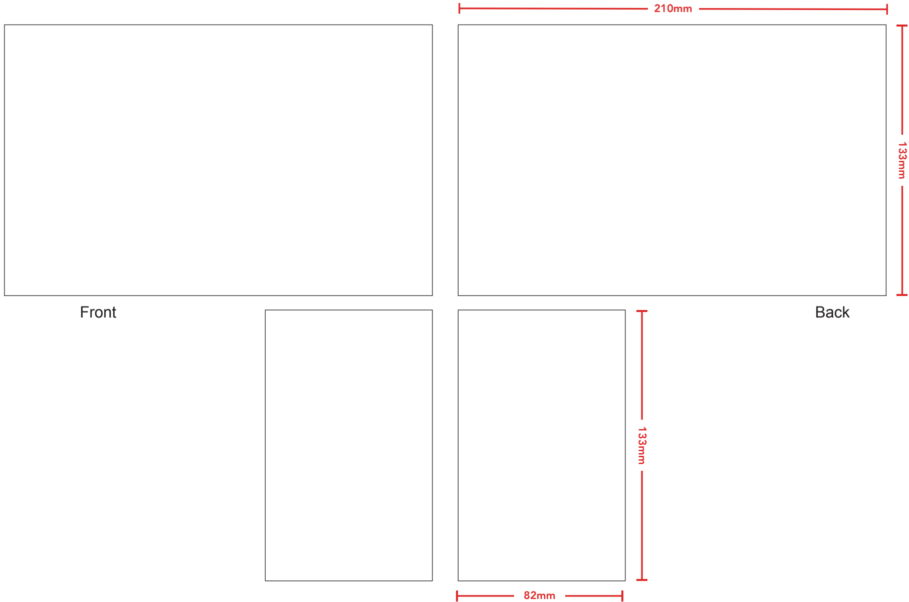
Left Gusset
